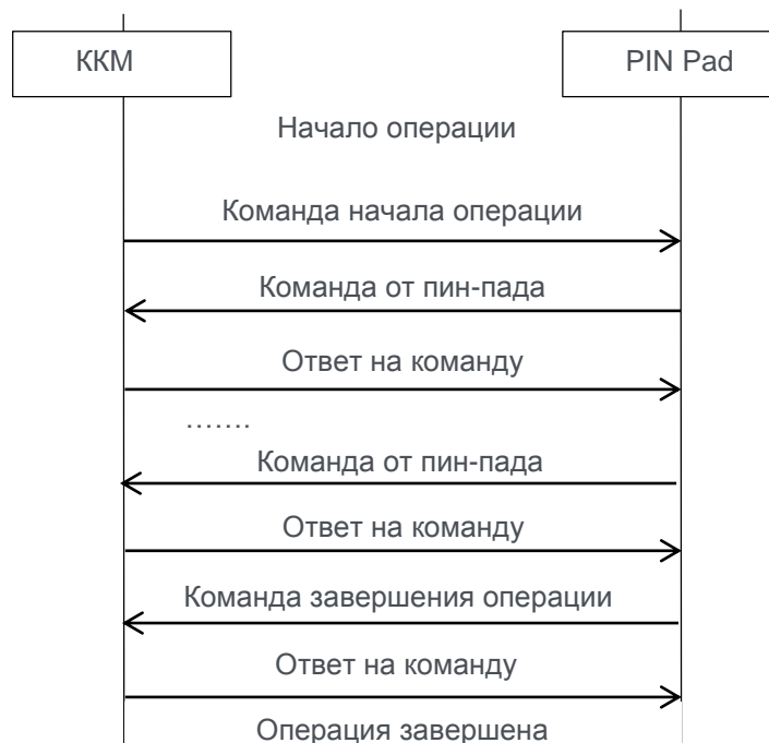
Рис. 10. Общая схема взаимодействия
