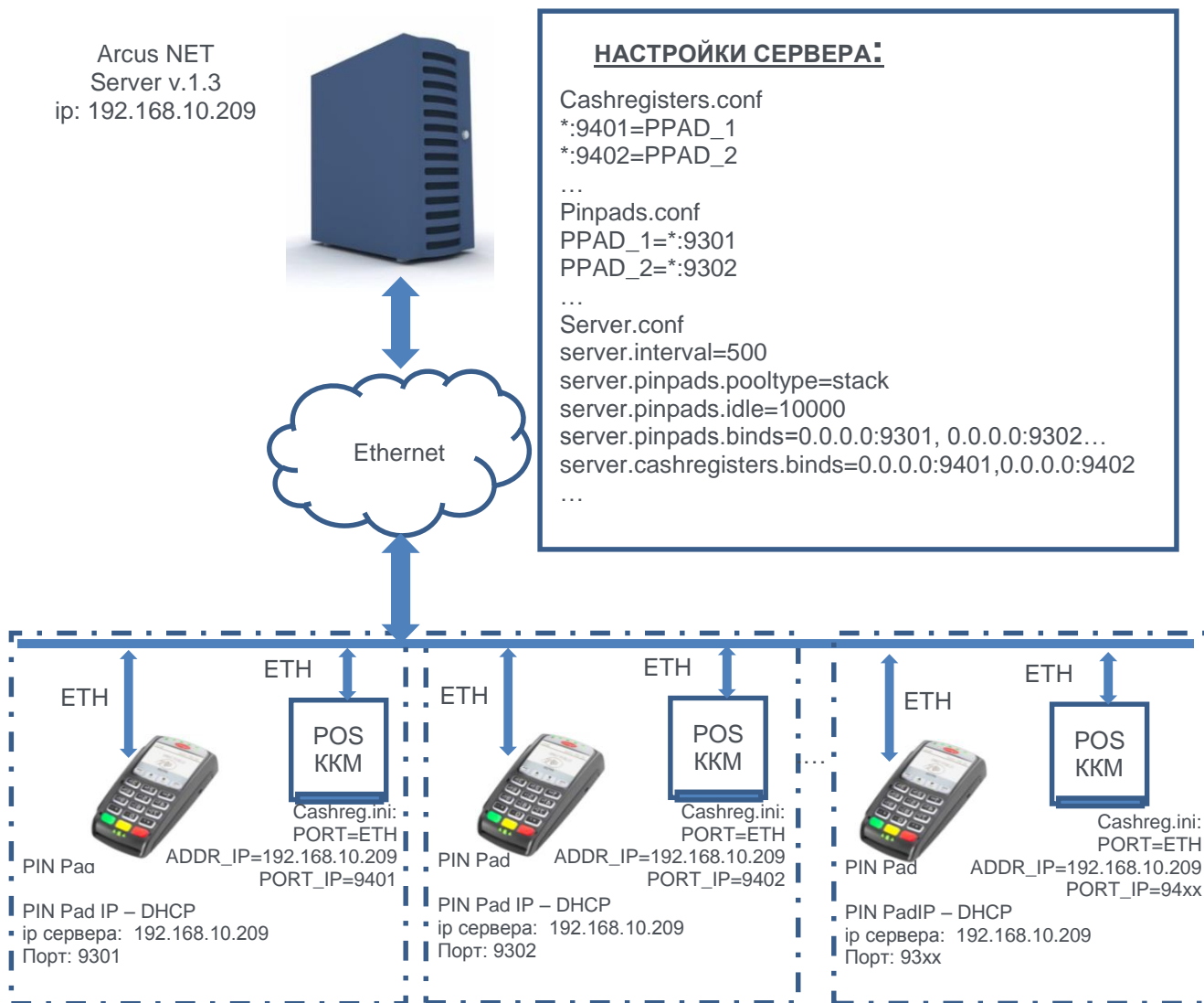
Рис. 13. Пример настройки сервера (более одной ККМ (ARCUS2) и более одного ПИН-пад)
