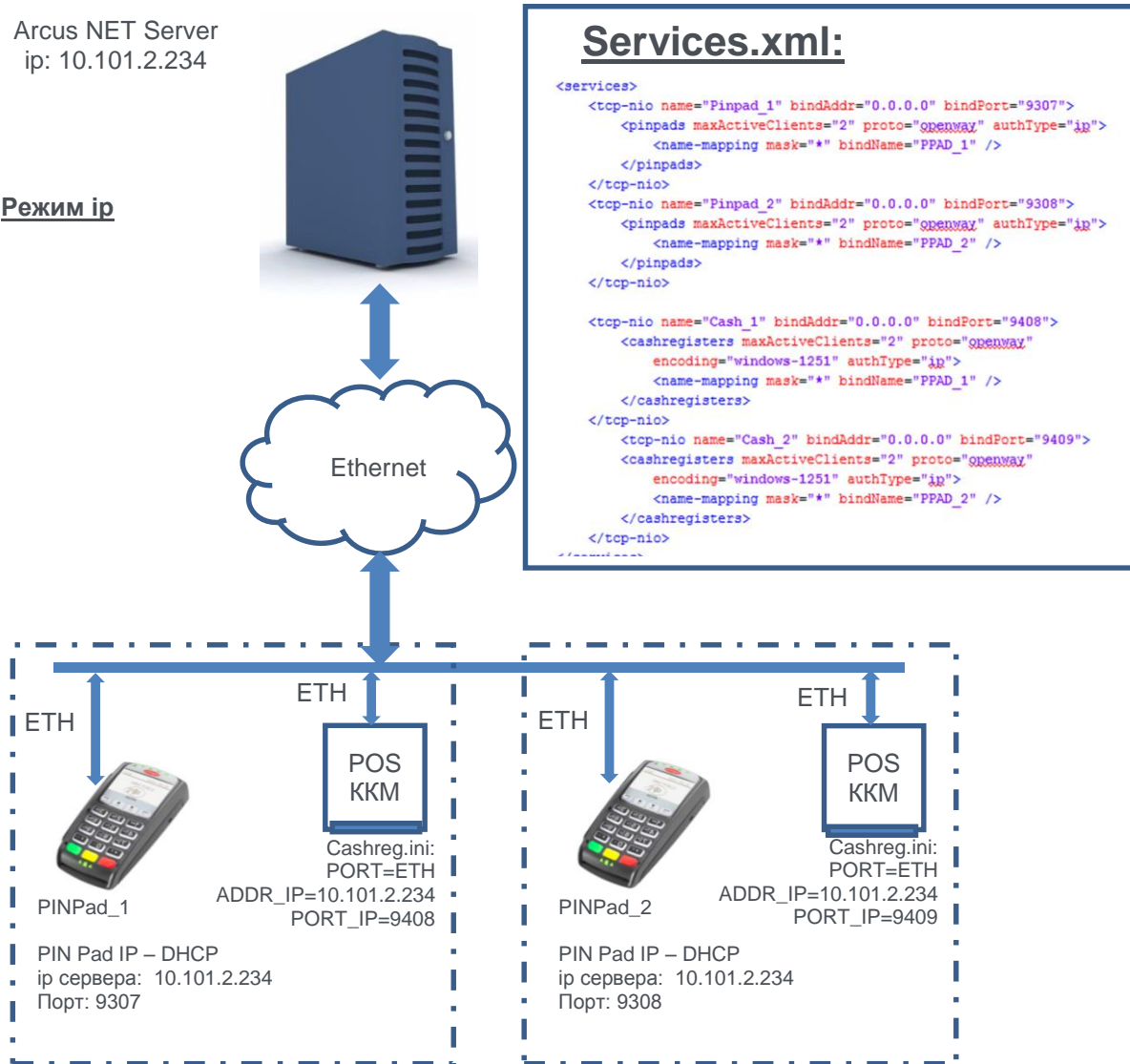
Рис. 16. Пример настройки Arcus NET Server v.2 – Режим IP
