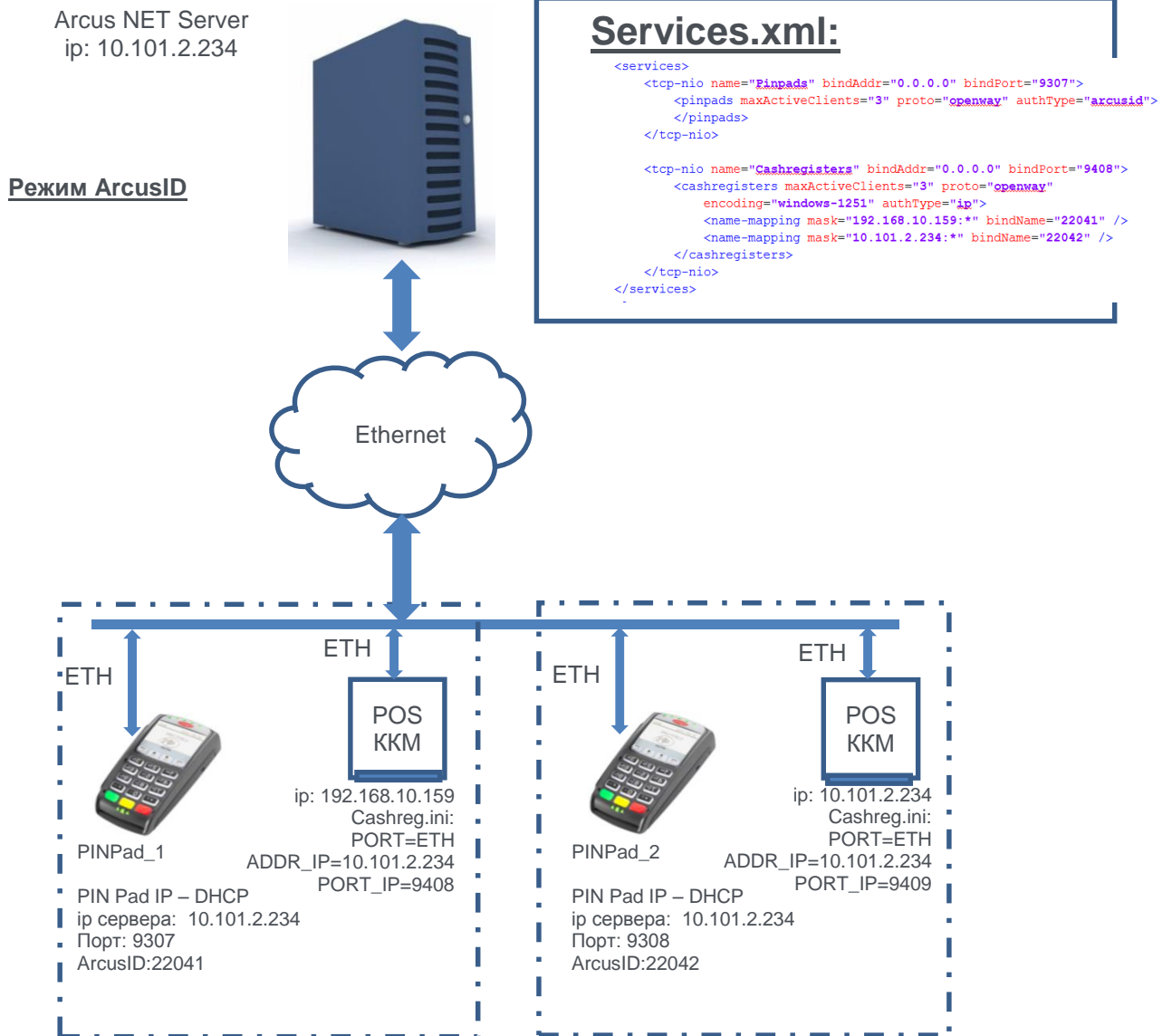
Рис. 15. Пример настройки Arcus NET Server v.2 – Режим Arcus ID
