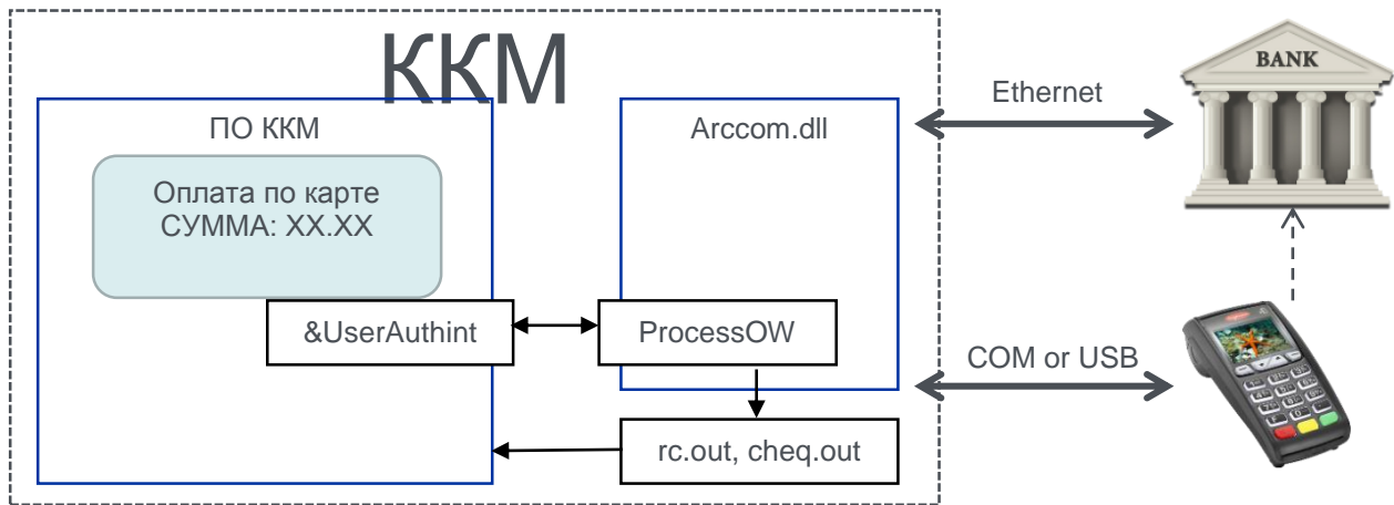
Рис. 3 Схема взаимодействия кассового ПО с модулем ArcCom.DLL
