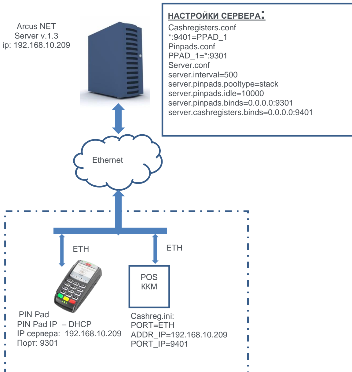
Рис. 12. Пример настройки сервера 1 ККМ-1 ПИН-пад
